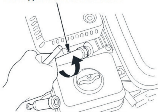
КЛЮЧ ДЛЯ СВЕЧИ ЗАЖИГАНИЯ
